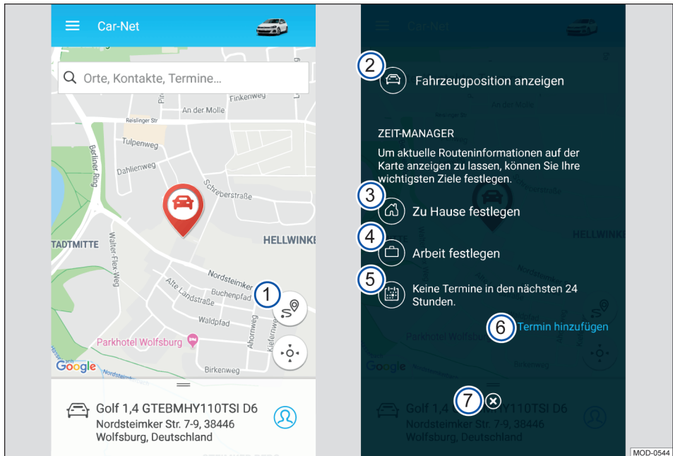
Abb. 7 Links: Startseite; rechts: zentrale Bedienoberfläche des Zeit-Managers.
